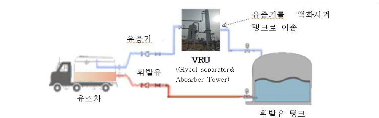
[그림 1] □○지사 VRU 설비 개념도
